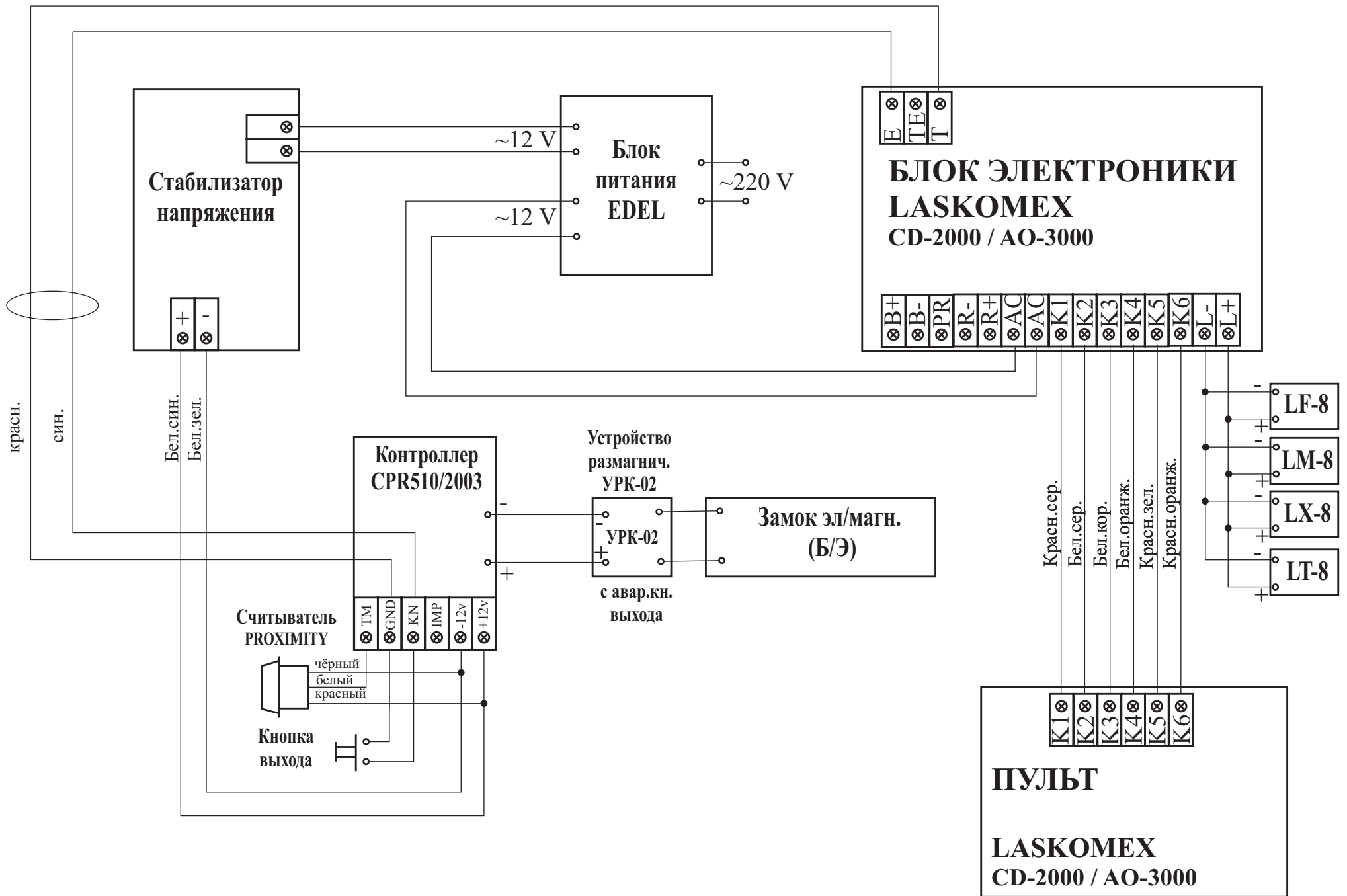
Монтажная схема домофона LASKOMEX с контроллером CPR510/2003
