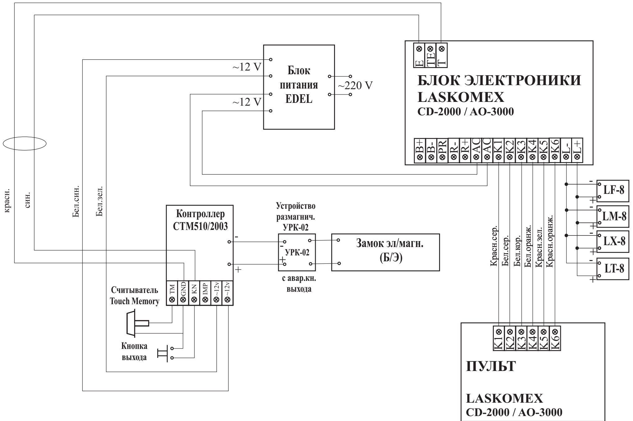
Монтажная схема домофона LASKOMEX с контроллером STM510/2003
