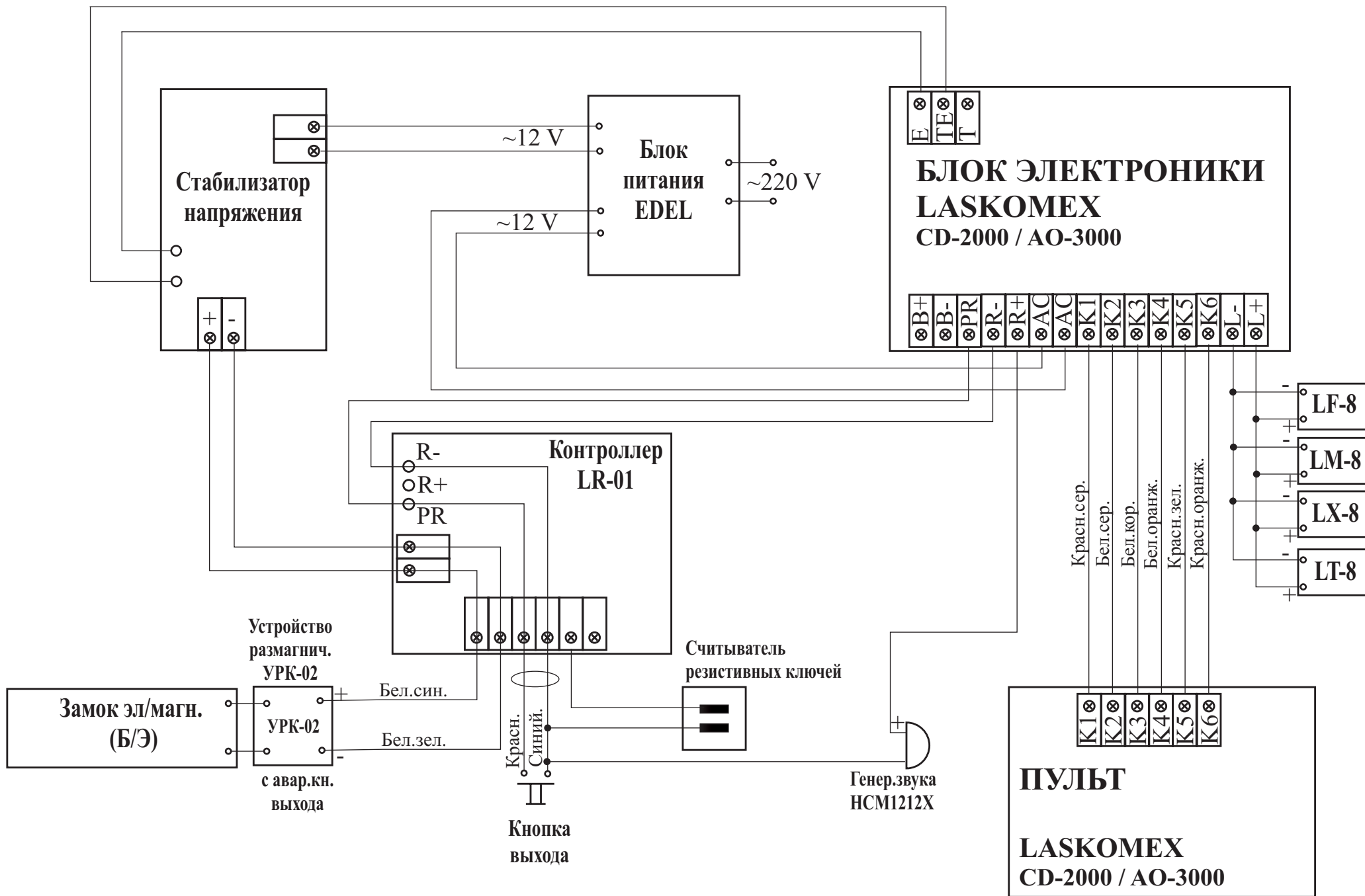
Монтажная схема домофона LASKOMEX с резистивным контроллером LR-01
