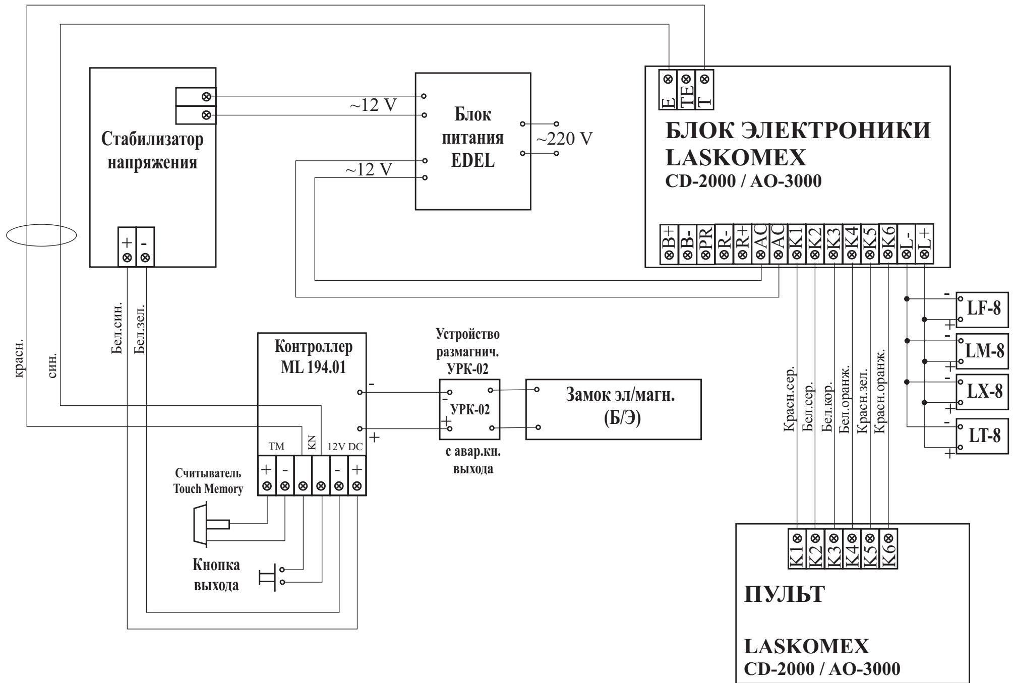
Монтажная схема домофона LASKOMEX с контроллером ML 194.01
